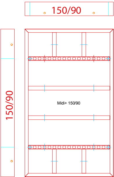
Midi + 150ht x 90
