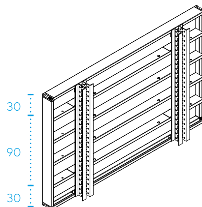
Panneau 240/150
