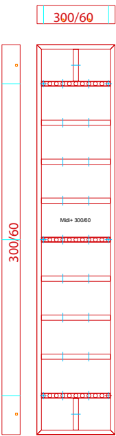
Midi + 300ht x 60
