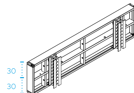
Panneau 240/60
