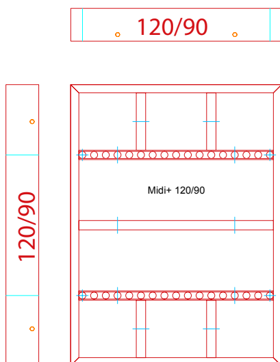
Midi + 120ht x 90
