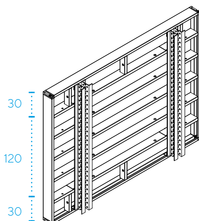
Panneau 240/180
