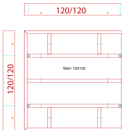
Midi + 120ht x 120
