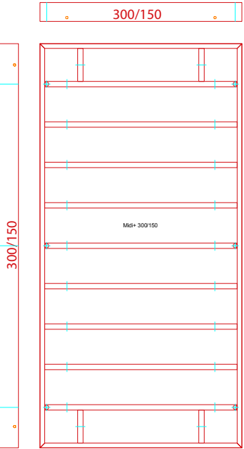
Midi + 300ht x 150
