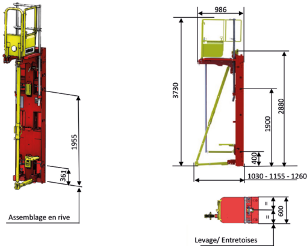
Panneau 280x60
