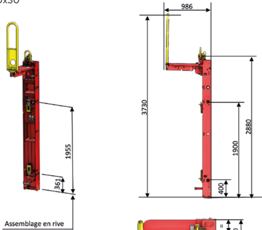
Panneau angle intérieur
