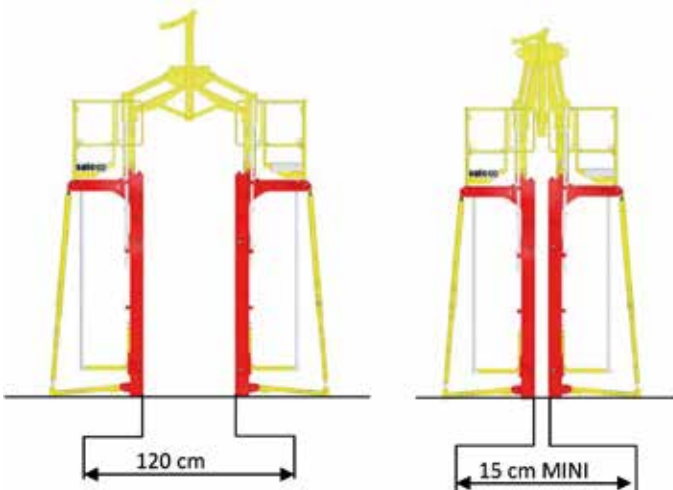
Portique ouverture 1m20
