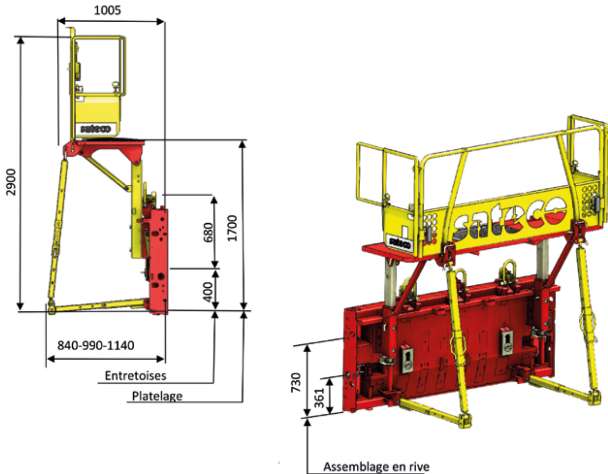
Sous-hausse hauteur 1000 et largeur 2400
