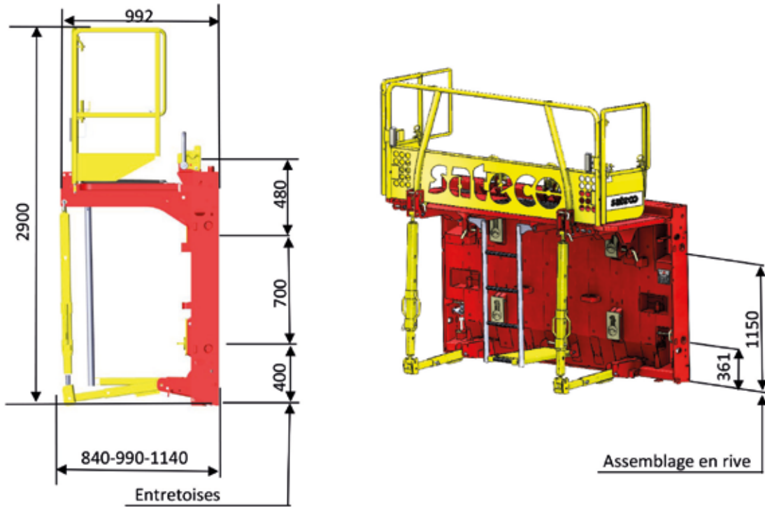
Sous-hausse hauteur 1500 et largeur 2400
