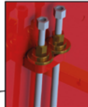
Stockage bas pour tiges entretoises
